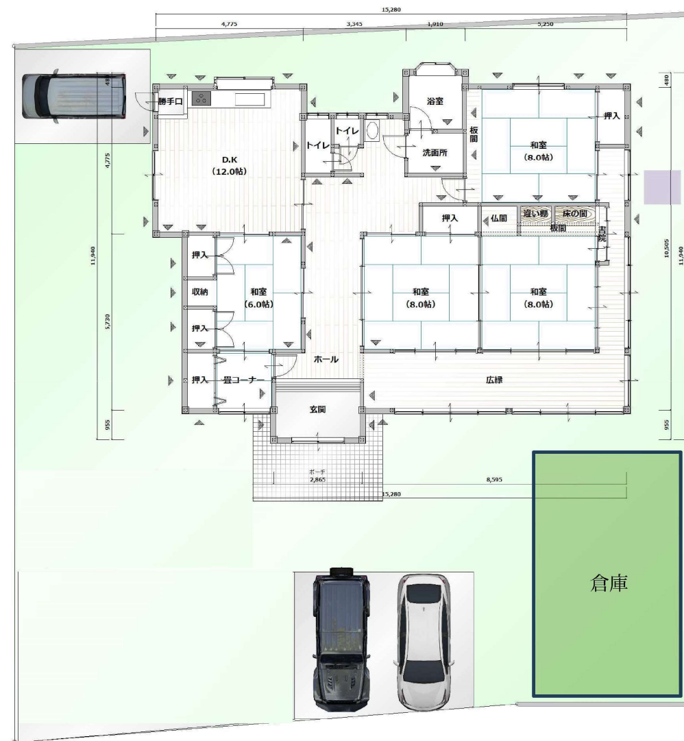
敷地配置図
